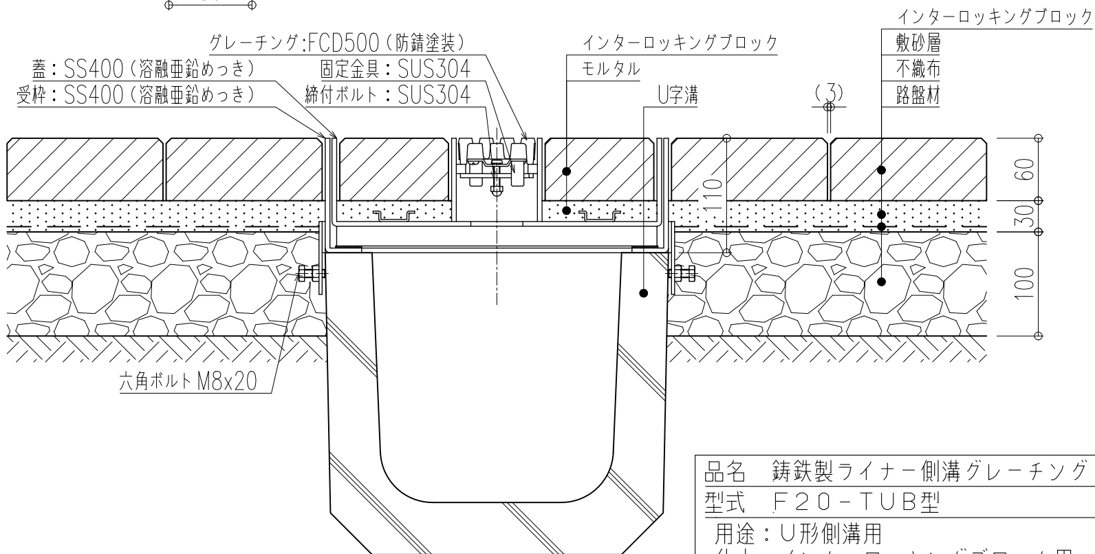
施工参考図
